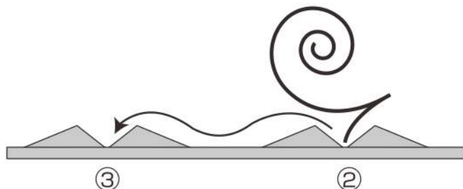
(II)手巻きゼンマイ、外端の拡大図
