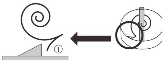
(I)手巻きゼンマイ、外端の拡大図
